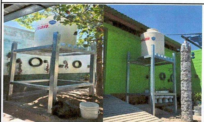
Foto 4: MEJORAMIENTO A INSTALACIÓN DE DEPÓSITOS DE AGUA
